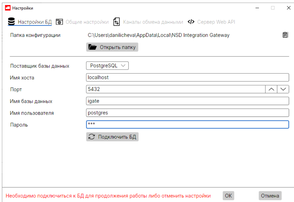
Рисунок 13. Настройки БД. PostgreSQL
