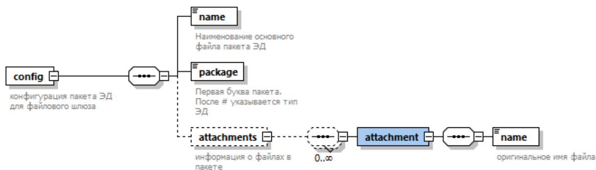
Рисунок 19. Структура файла config.xml
