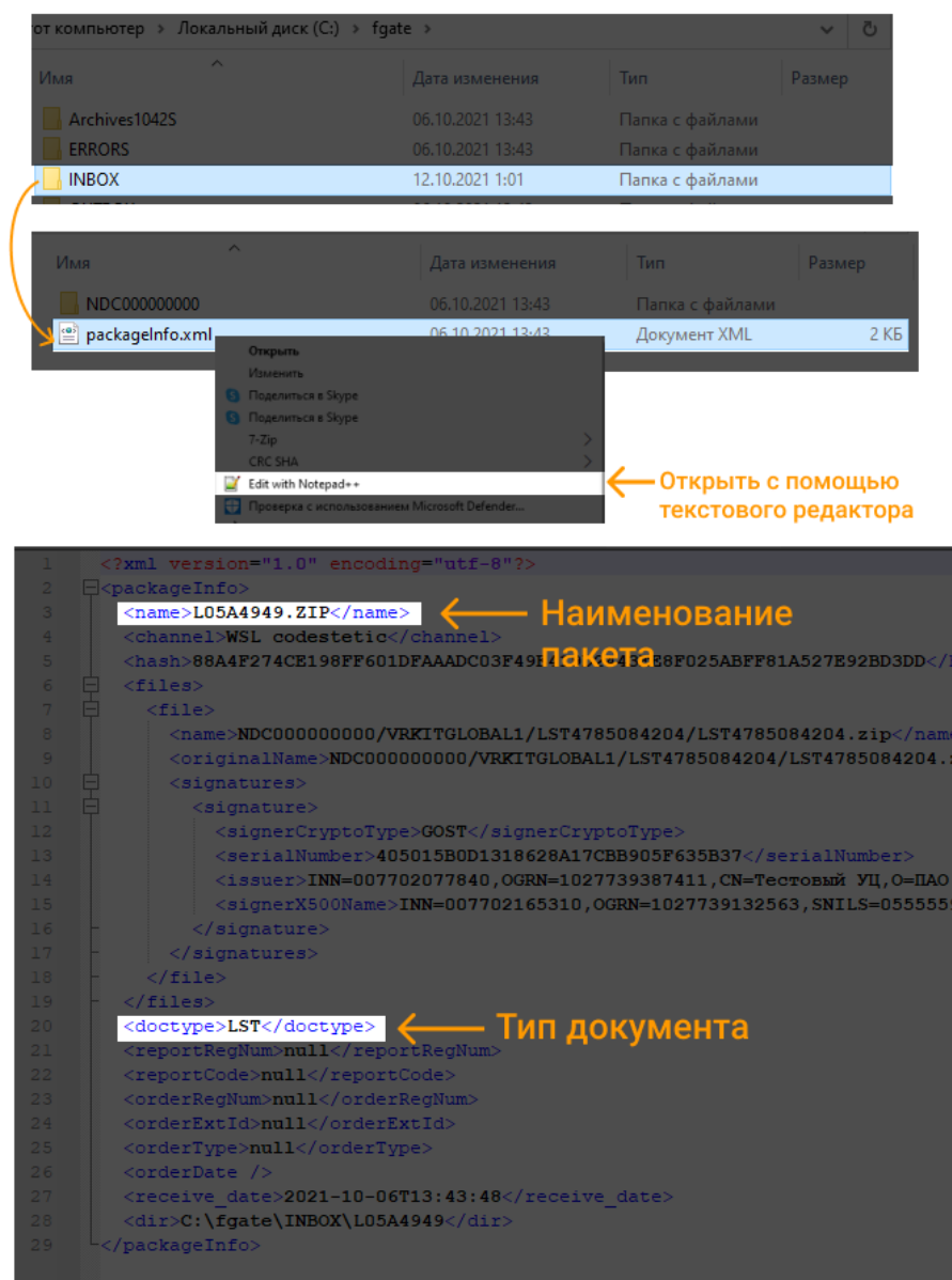
Рисунок 21. Просмотр информации в packageInfo.xml
